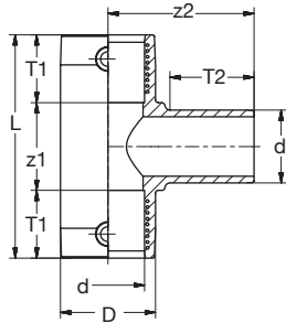
BR PE100 E-T-Stück 90° mit Schweißstutzen SDR11 schwarz BR PE100 E-Tee 90° with spigot SDR11 black
