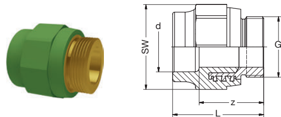
BR PP-R- RG/LFB Verschraubung Schraubteil flachdichtend grün BR PP-R- Bronze/LFB Union Srew-part flat-sealing green
