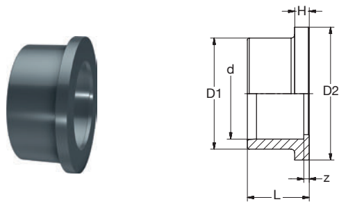
BR PVC-U Bundbuchse glatt grau
