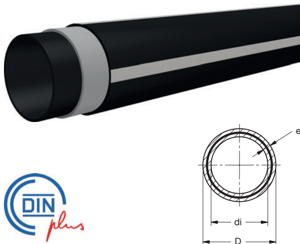
BR PE100 Druckrohr BLACKTECplus SDR11 1,6MPa schwarz 5m BR PE100 Pressure pipe BLACKTECplus SDR11 1.6MPa black 5m
