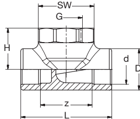
BR PP-R-LFB Ventil Geradsitz Unterteil IG-zyl grün BR PP-R-LFB Valve straight bottom part female-thread-cyl green
