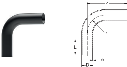
BR PE100 Rohrbogen 90° nahtlos lang SDR11 schwarz
