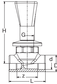
BR PP-R-Ms Ventil Geradsitz UP Drehgriff grün BR PP-R-Brass Valve straight concealed handle bar green
