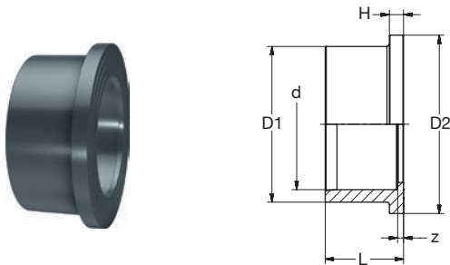
BR PVC-U Bundbuchse gerillt grau
