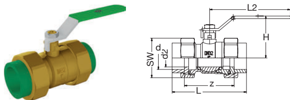
BR PP-RCT Kugelhahn-Ms verschraubt Runddichtring-EPDM 20°C/1,0MPa grün BR PP-RCT Ball valve Brass with union-nuts O-Ring-gasket-EPDM 20°C/1.0MPa green
